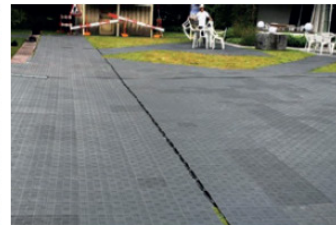
Bild 3: Falsch! Verlegung ohne Dehnungsfugen, Boden wellt sich bei Sonneneinstrahlung
