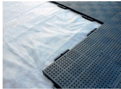
Bild 1: Verlegung ohne Geovlies, Rasen wird geschont und wächst sogar durch
